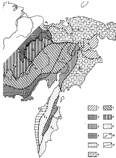
Рис.1. Схема физико-географического районирования
